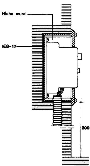
Sección
