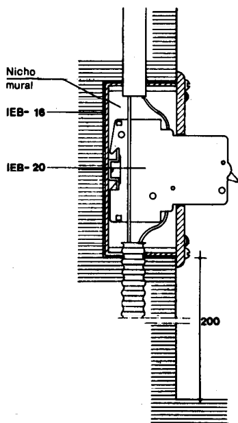
Sección
